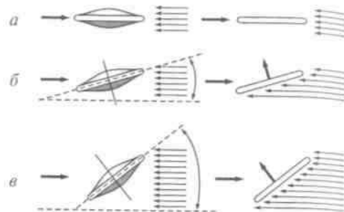
Рис. 65. Возникновение подъемной силы у летящего диска: a — прямой удар; б — косой удар с нормальным положением диска; в — косой удар с повышенным углом атаки
