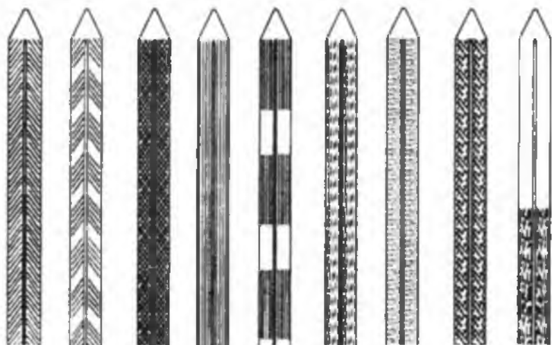
Рис. 39. Структурные рисунки, наносимые на скользящую поверхность лыж
