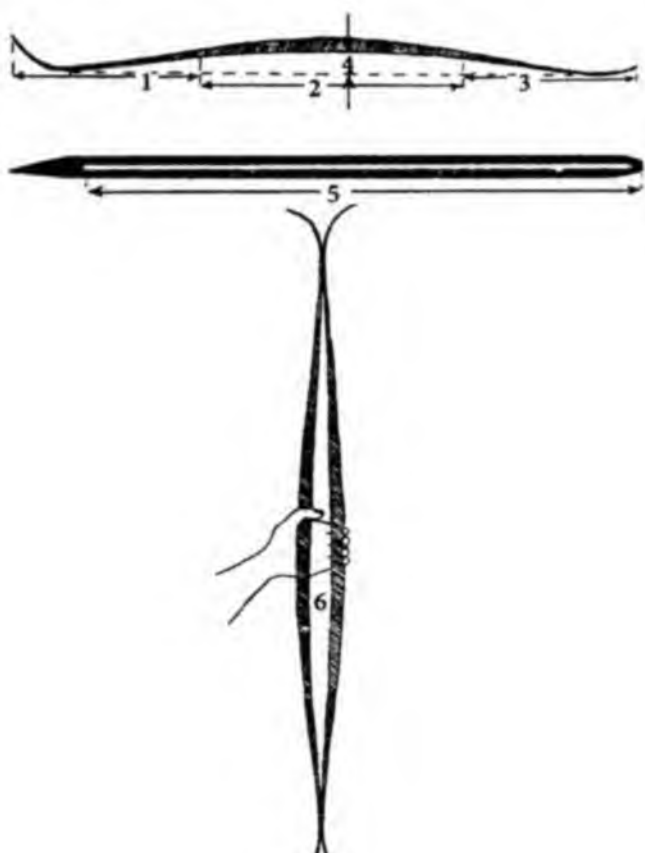
Рис. 30. Части скользящей лыжи: носочная -1, колодка -2, пяточная -3, весовой прогиб -4, желобок -5; простейший способ определения жесткости лыж -6
